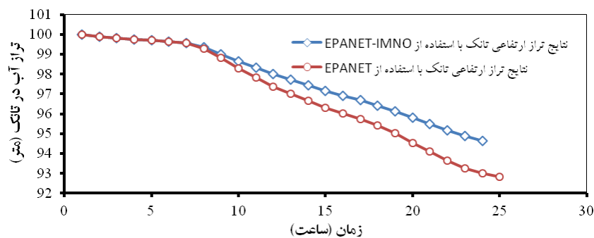
شکل ۱- مقایسه نتایج تراز ارتفاعی تانک با دو نوع شبیه ساز EPANET
